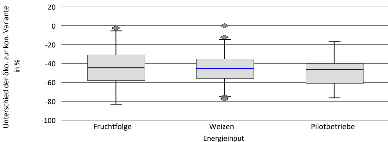
Abbildung 8.8 Relative Unterschiede zwischen der ökologischen und konventionellen Landwirtschaft hinsichtlich des Energieinputs
