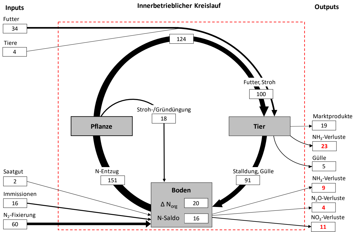
Abbildung 8.1 Stickstoffkreislauf (N-Flüsse in kg/ha) eines ökologischen Gemischtbetriebs mit Rinderhaltung
